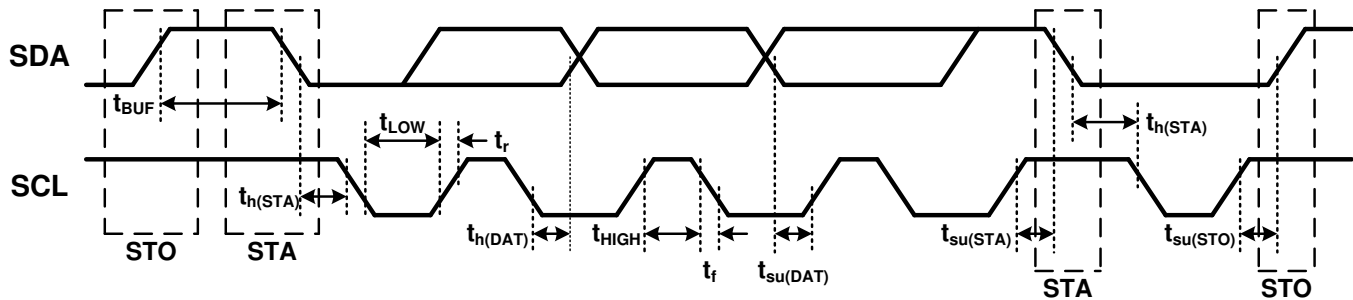
图 1. I²C Timing Diagram
