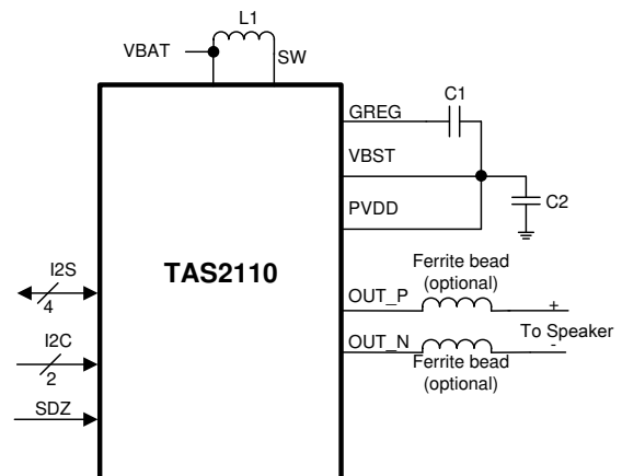
简化原理图
