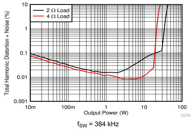
图 7-8. THD+N vs Power
