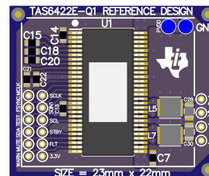
PCB 区域
