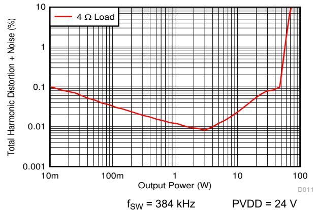
图 7-10. THD+N vs Power
