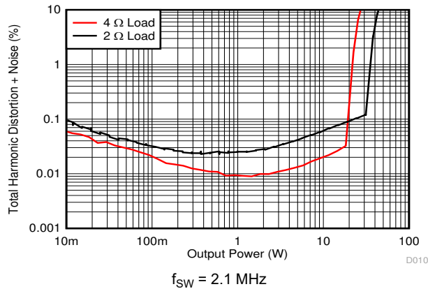
图 7-9. THD+N vs Power
