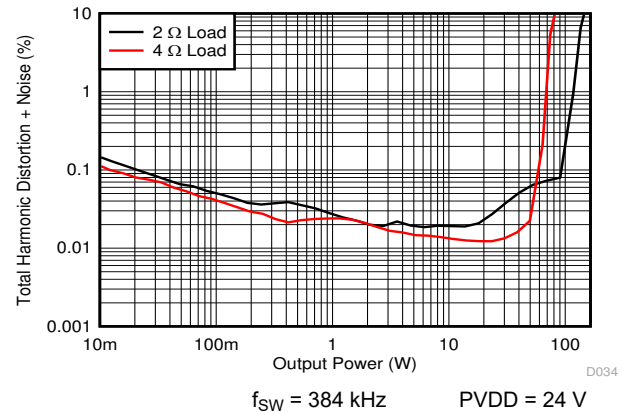
图 7-28. PBTL THD+N vs Power
