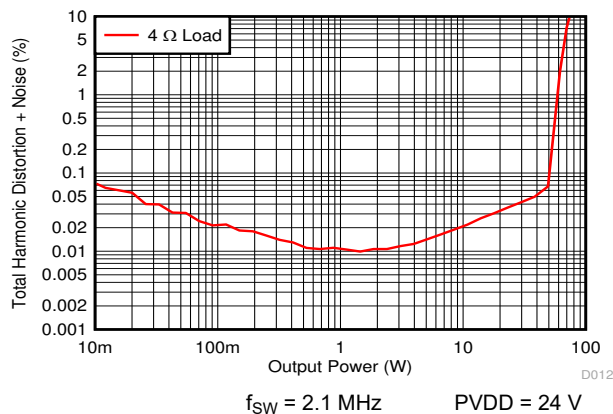
图 7-11. THD+N vs Power
