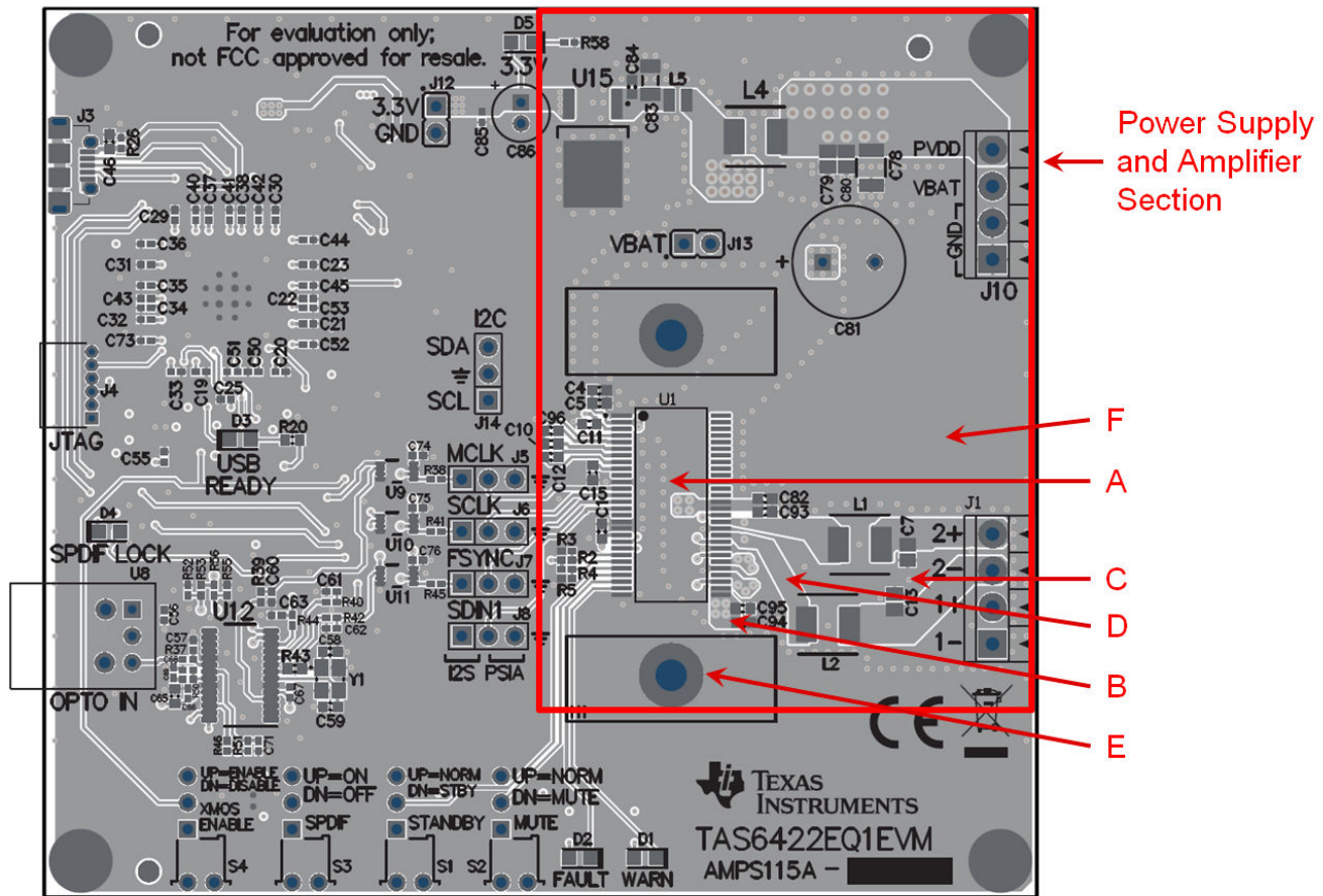
图 12-1. EVM Layout
