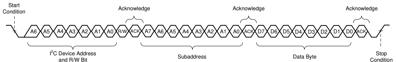
图 9-11. Random Write Transfer
