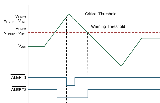
图 45. Comparator Hysteresis Behavior (INA302-Q1)
