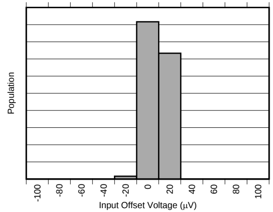
图 2. Input Offset Voltage Distribution (INA30xA2-Q1)
