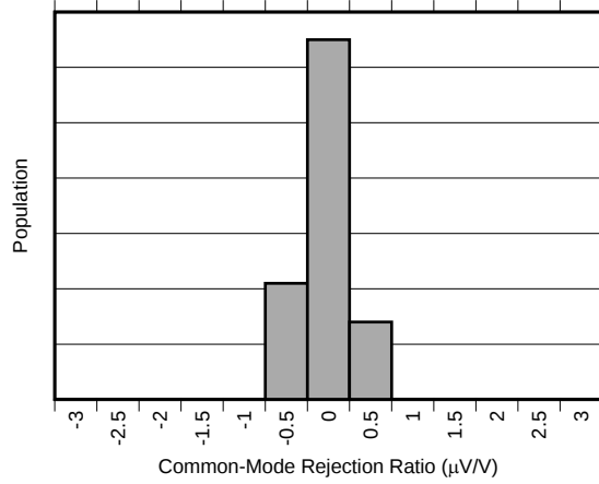
图 7. CMRR Distribution (INA30xA3-Q1)
