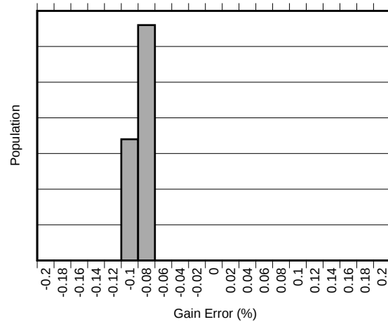
图 10. Gain Error Distribution (INA30xA1-Q1)
