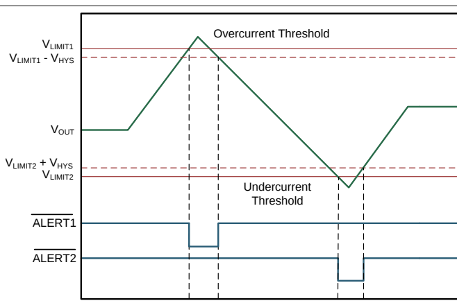
图 46. Comparator Hysteresis Behavior (INA303-Q1)
