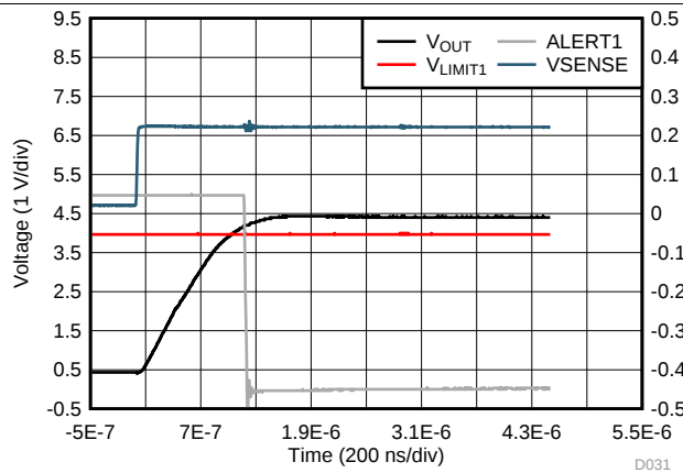
图 31. Comparator 1 Total Propagation Delay (INA30x-Q1)
