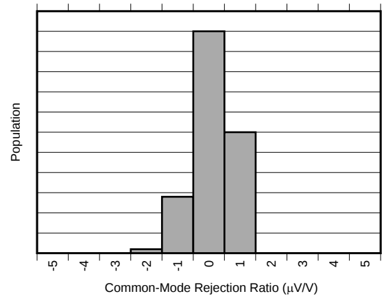
图 6. CMRR Distribution (INA30xA2-Q1)
