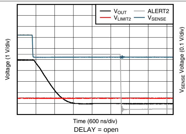
图 32. Comparator 2 Total Propagation Delay (INA303-Q1)
