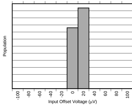
图 1. Input Offset Voltage Distribution (INA30xA1-Q1)
