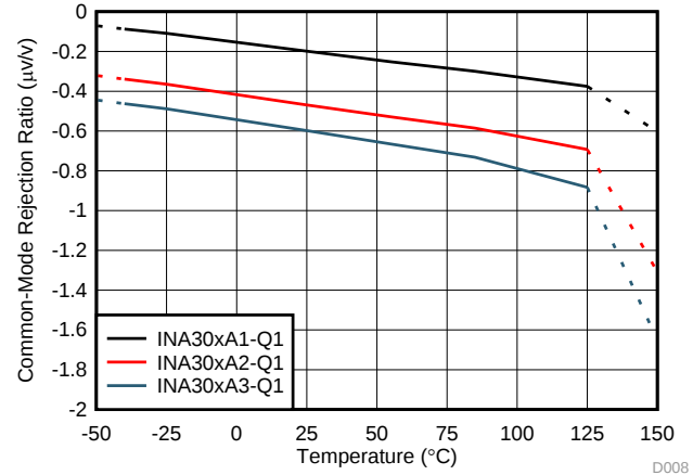
图 8. CMRR vs Temperature
