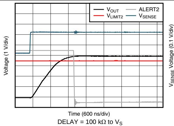
图 33. Comparator 2 Total Propagation Delay (INA303-Q1)
