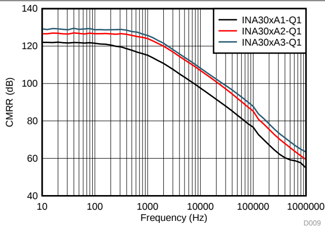
图 7. CMRR Distribution (INA30xA3-Q1)
