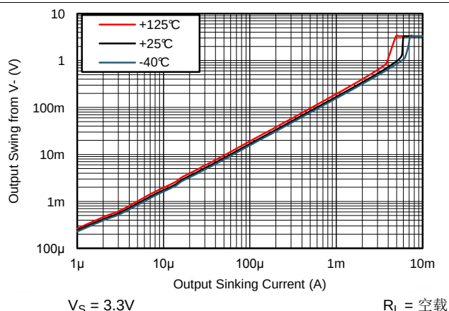
图 16. 输出摆幅与灌电流间的关系, 3.3V
