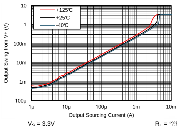
图 15. 输出摆幅与拉电流间的关系, 3.3V
