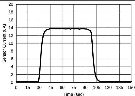
图 40. 计算出的传感器电流
