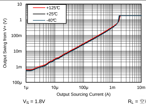
图 13. 输出摆幅与拉电流间的关系, 1.8V
