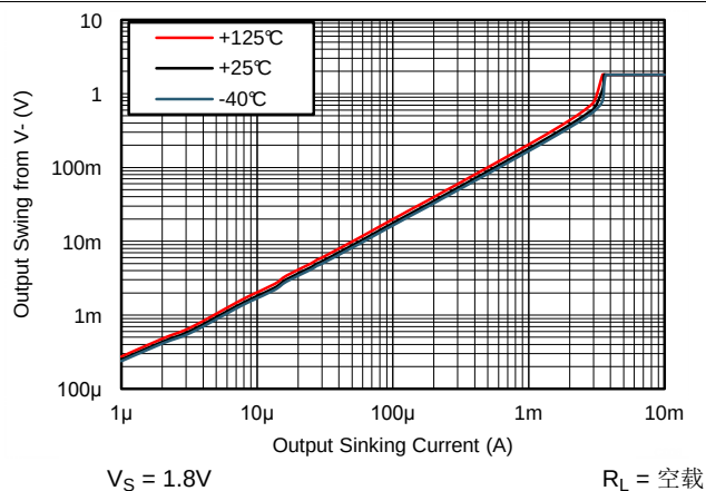
图 14. 输出摆幅与灌电流间的关系, 1.8V
