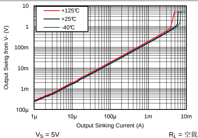
图 18. 输出摆幅与灌电流间的关系, 5V
