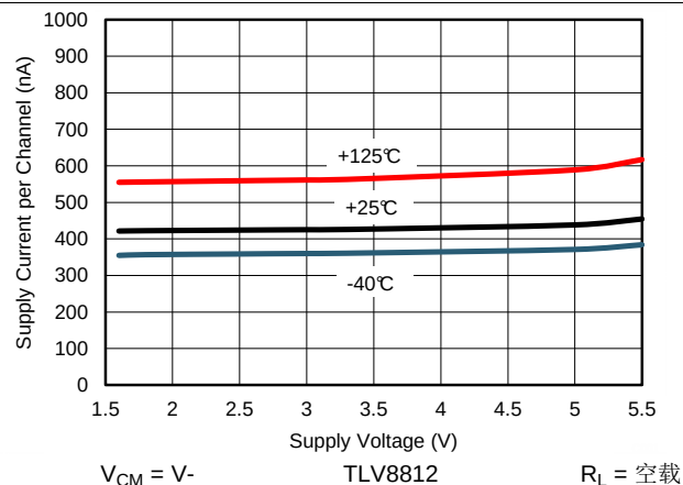
图 2. 电源电流与电源电压间的关系, TLV8812
