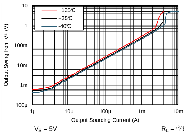
图 17. 输出摆幅与拉电流间的关系, 5V
