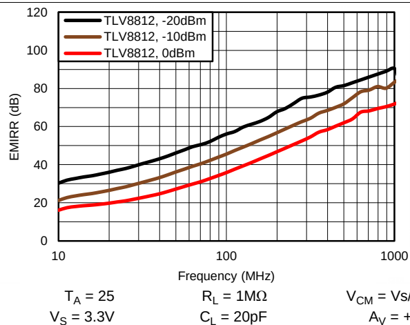
图 36. EMIRR 性能
