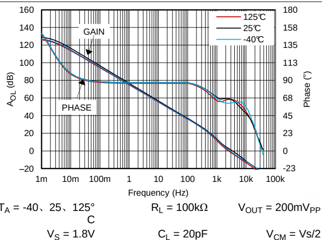
图 35. 开环增益和相位, 1.8V, 100kΩ 负载
