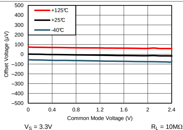
图 4. 典型偏移电压与共模电压间的关系
