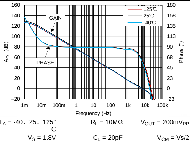
图 31. 开环增益和相位, 1.8V, 10MΩ 负载
