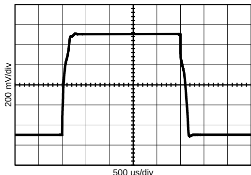
图 19. 小信号脉冲响应, 1.8V
