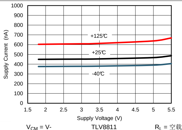
图 1. 电源电流与电源电压间的关系, TLV8811
