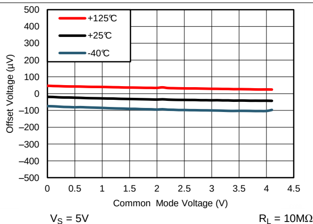
图 5. 典型偏移电压与共模电压间的关系
