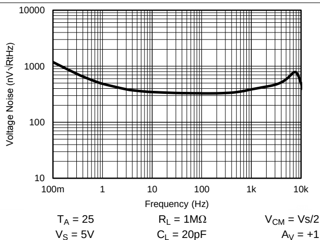
图 34. 输入电压噪声与频率间的关系
