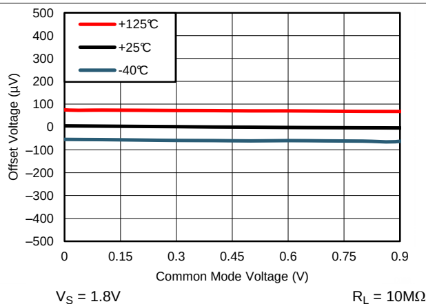
图 3. 典型偏移电压与共模电压间的关系
