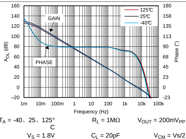
图 33. 开环增益和相位, 1.8V, 1MΩ 负载
