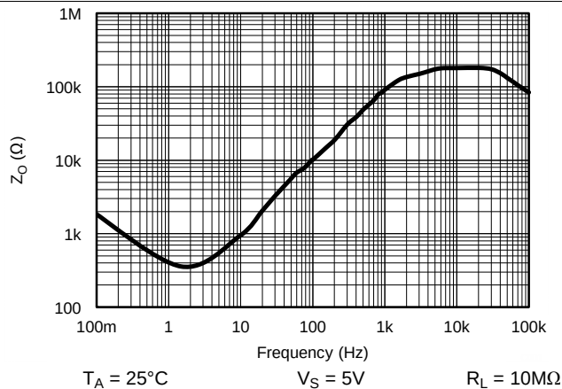
图 32. 开环输出阻抗
