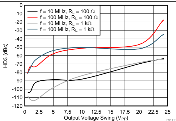
图 14. HD3 vs Output Swing
