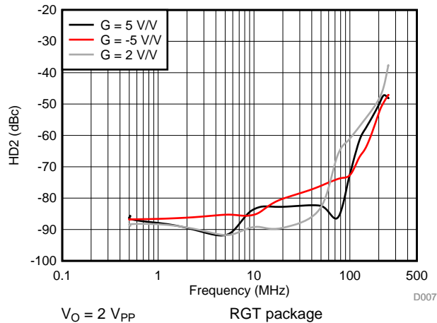
图 9. HD2 vs Frequency
