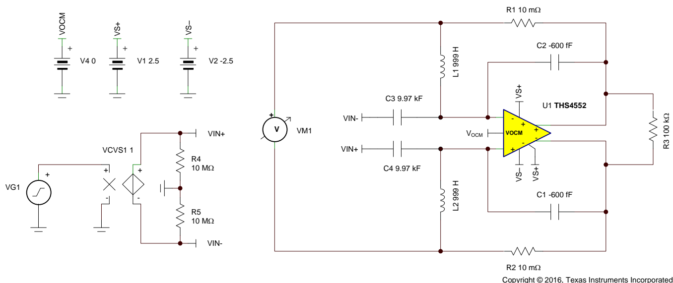
图 102. 开环增益和相位 TINA-TI™ 仿真设置
