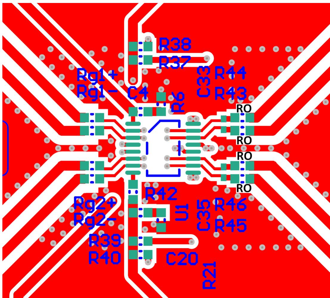
图 99. Example Layout
