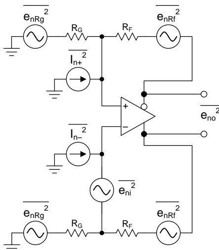
图 77. FDA Noise Analysis Circuit
