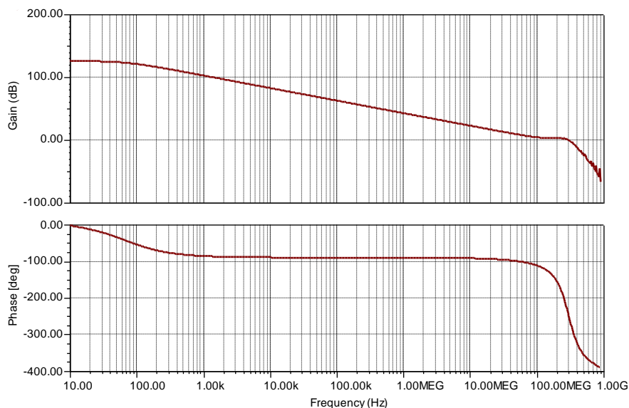
图 103. 开环增益和相位仿真结果
