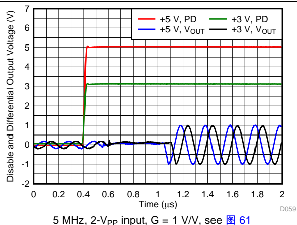
图 59. \overline{\text{PD}} Turn-On Waveform
