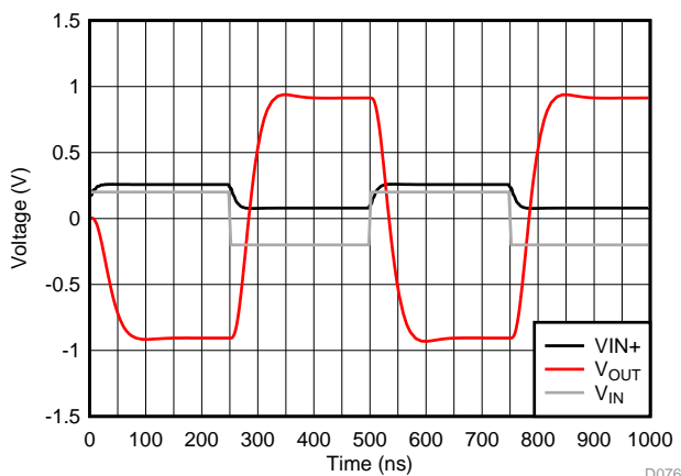
图 97. Time-Domain Waveform
