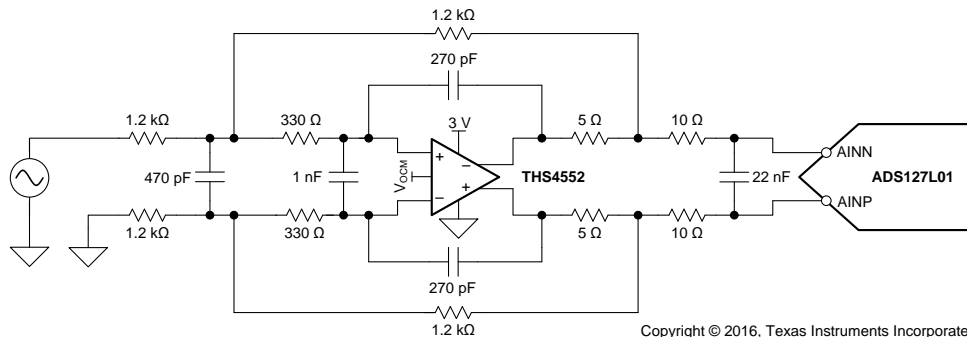
简化原理图：1V/V 增益、单端输入转差分输出、500kHz、 ADS127L01 多反馈滤波器接口（两条通道之一）
