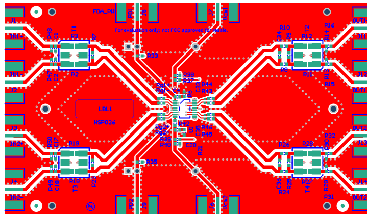
图 100. THS4552PWEVM Top Layer
