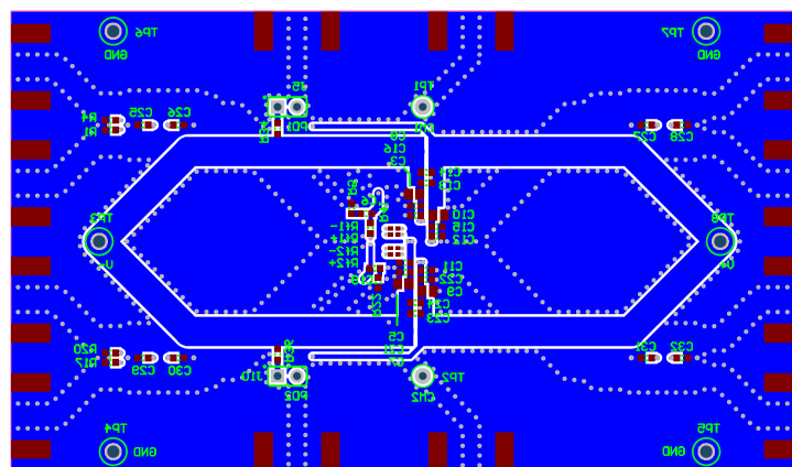
图 101. THS4552PWEVM Bottom Layer
