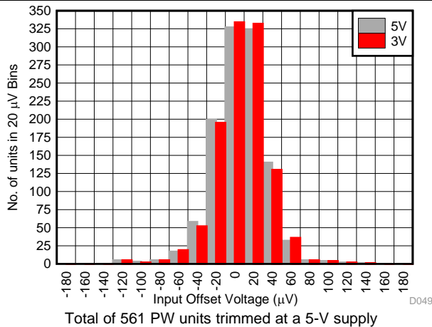
图 49. Input Offset Voltage ( V_{\text{IO}} )
