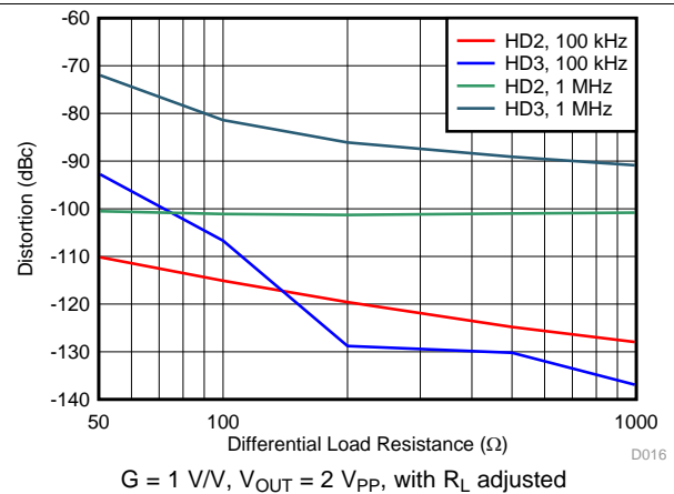
图 16. Harmonic Distortion vs R_L
