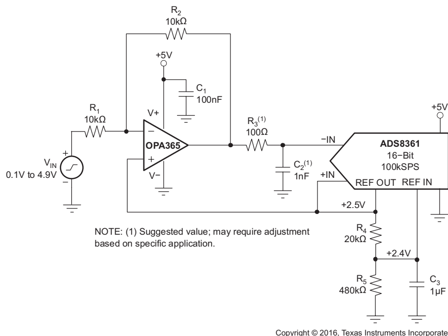
图 31. 驱动 ADS8361
