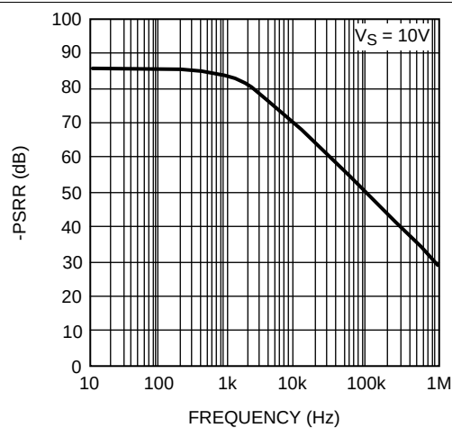
图 36. -PSRR 与频率间的关系
