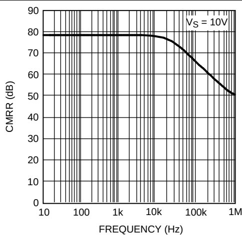
图 34. CMRR 与频率间的关系
