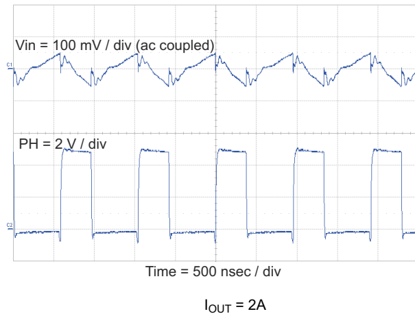
Figure 8-8. Input Ripple
