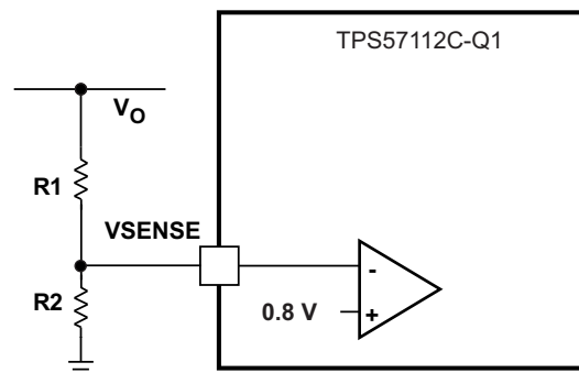
图 21. Voltage-Divider Circuit
