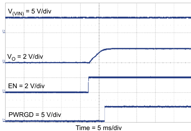
图 43. Power-Up V_O , EN
