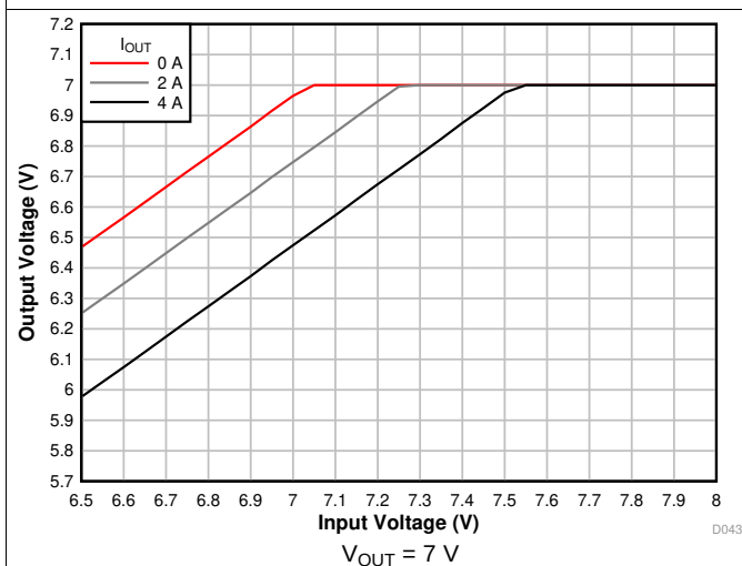
图 35. Voltage Dropout
