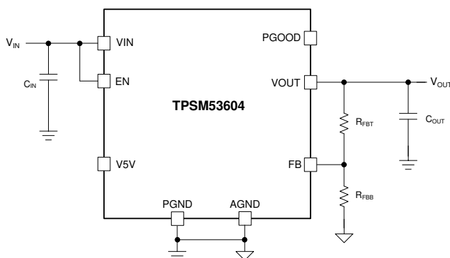
简化原理图
