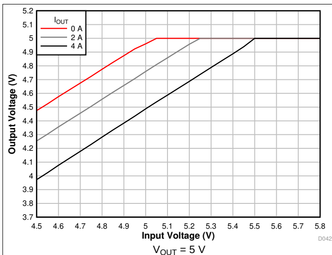
图 33. Voltage Dropout
