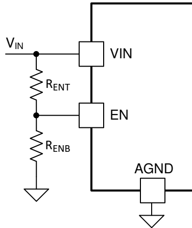
图 29. Adjustable UVLO
