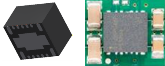
RLF 封装和典型布局
