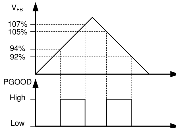
图 30. Power-good Flag
