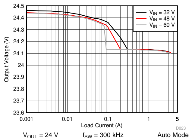
图 47. LM76003-Q1 Load and Line Regulation
