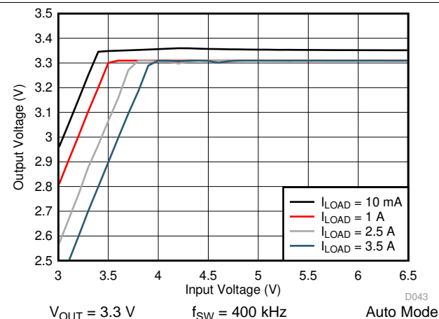
图 51. LM76003-Q1 Dropout Curve
