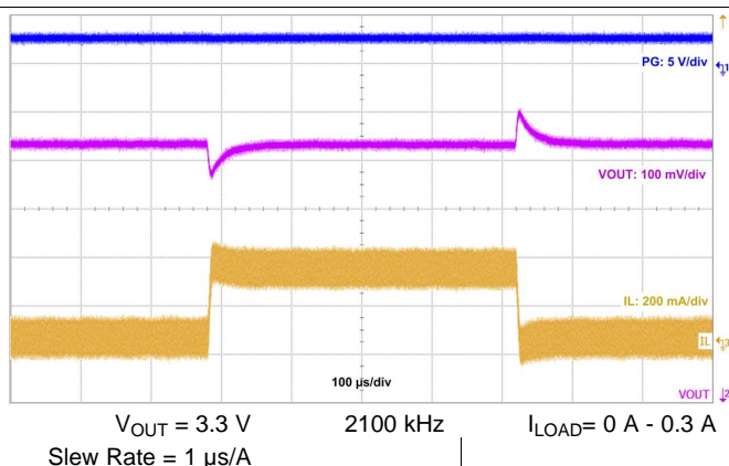
图 39. Load Transient
