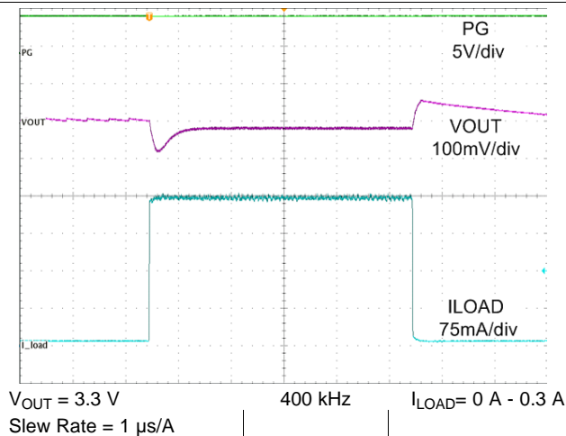
图 33. Load Transient
