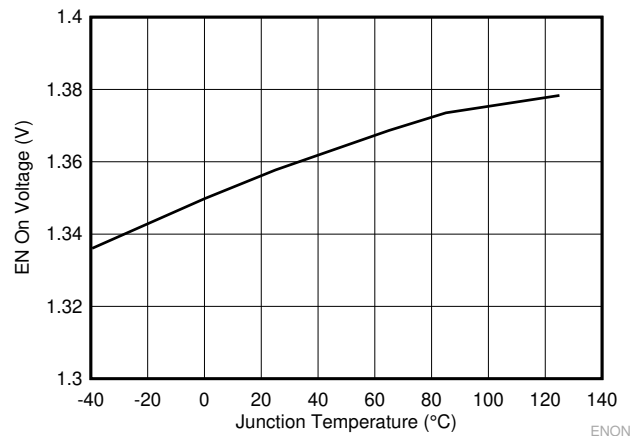
图 7-4. EN Pin EN On Voltage vs Junction Temperature
