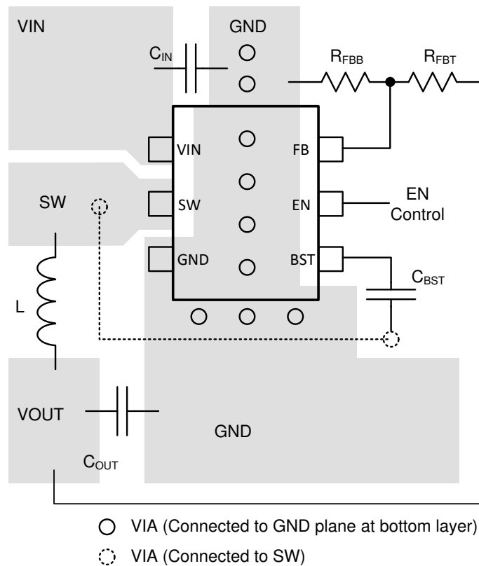
图 11-1. TPS563207S Layout
