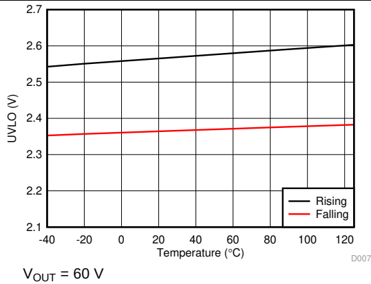
图 7. Vin UVLO
