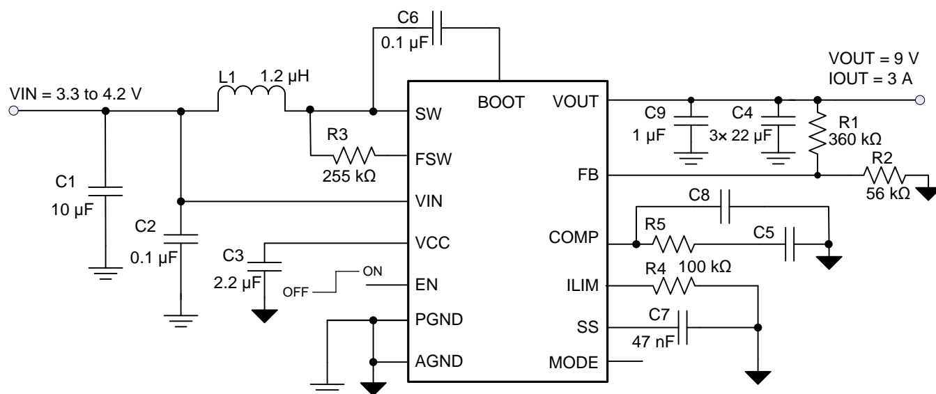
图 12. TPS61088 3.3 V to 9-V/3-A Output Converter
