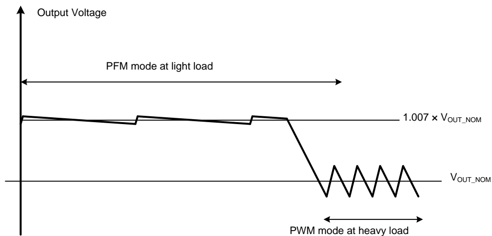
图 11. PFM Mode Diagram
