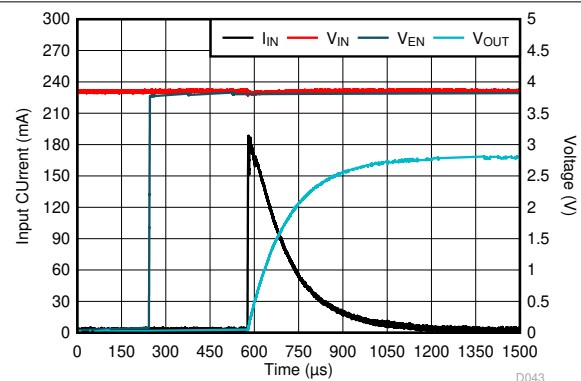
图 6-82. Startup
