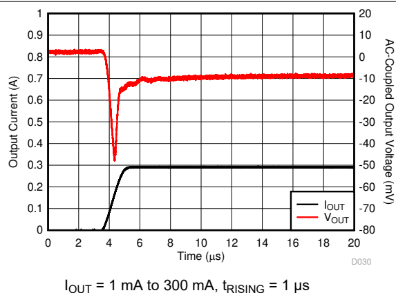
图 6-51. Load Transient
