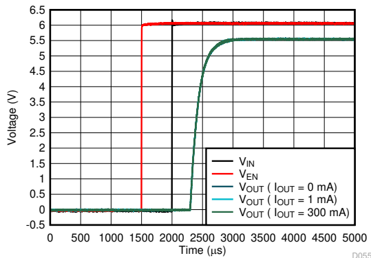
图 6-79. Startup
