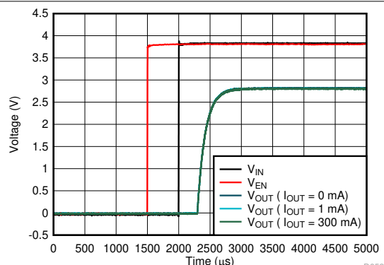
图 6-76. Startup
