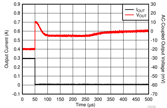
图 6-56. Load Transient
