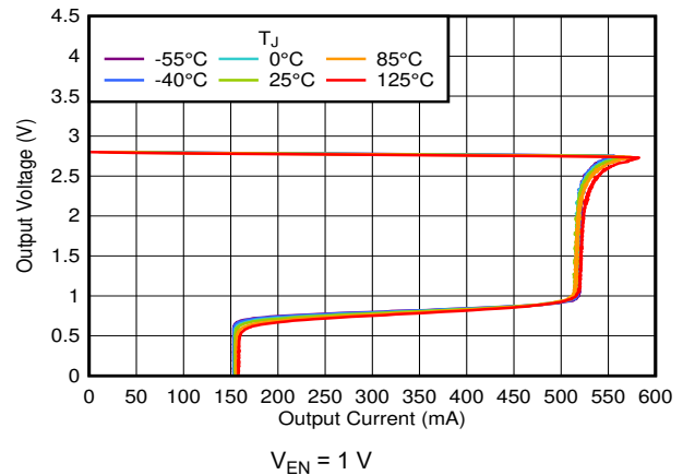
图 6-44. Current Limit
