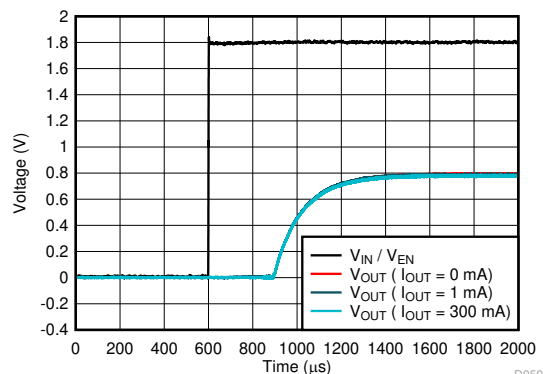
图 6-74. Startup
