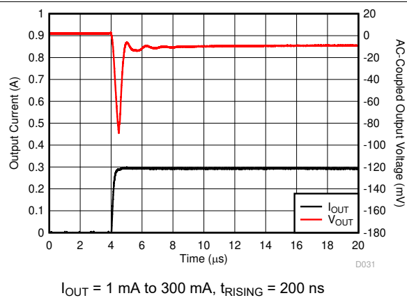
图 6-53. Load Transient
