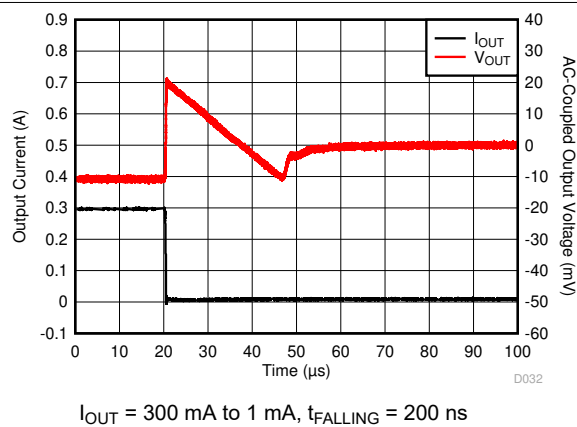
图 6-54. Load Transient
