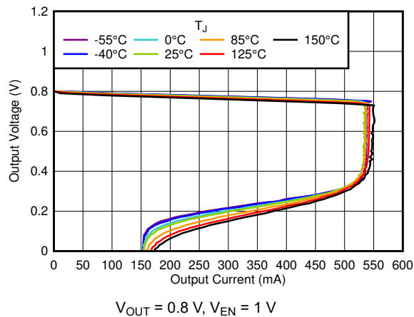
图 6-45. Current Limit
