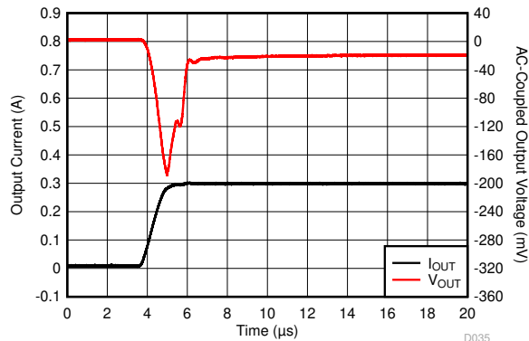
图 6-55. Load Transient
