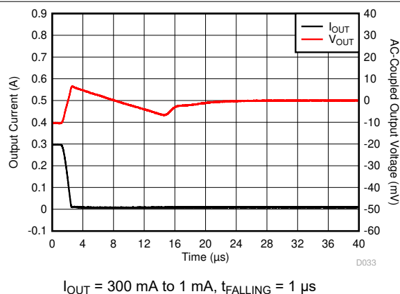
图 6-52. Load Transient
