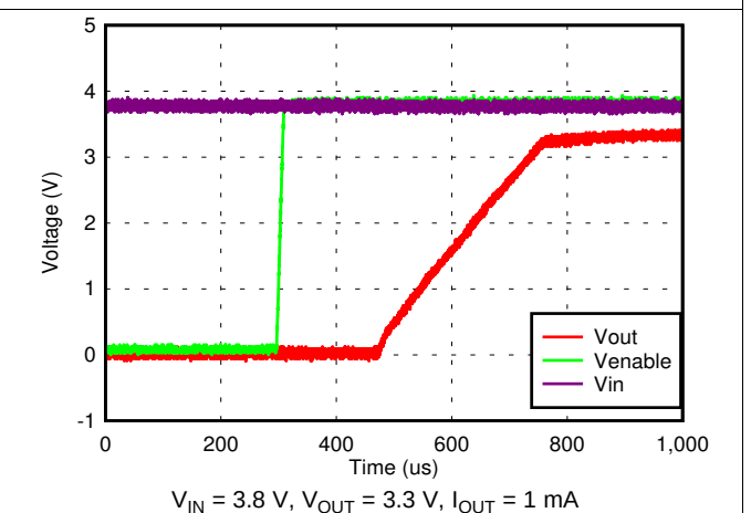
图 24. Startup With EN
