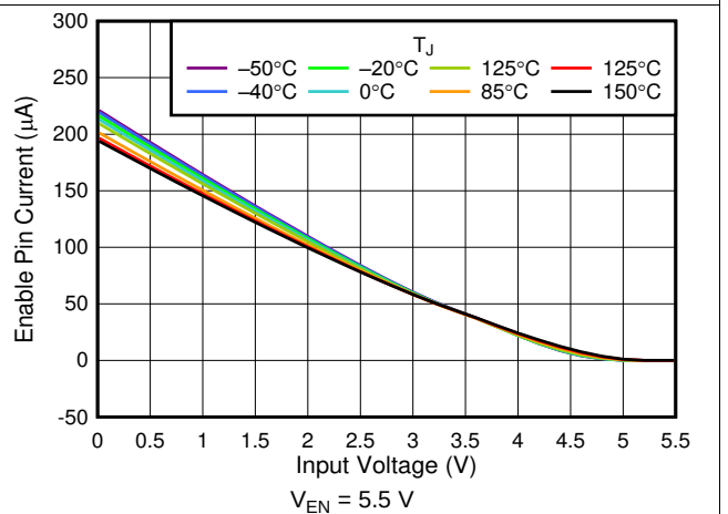
图 16. I_{EN} vs V_{IN}
