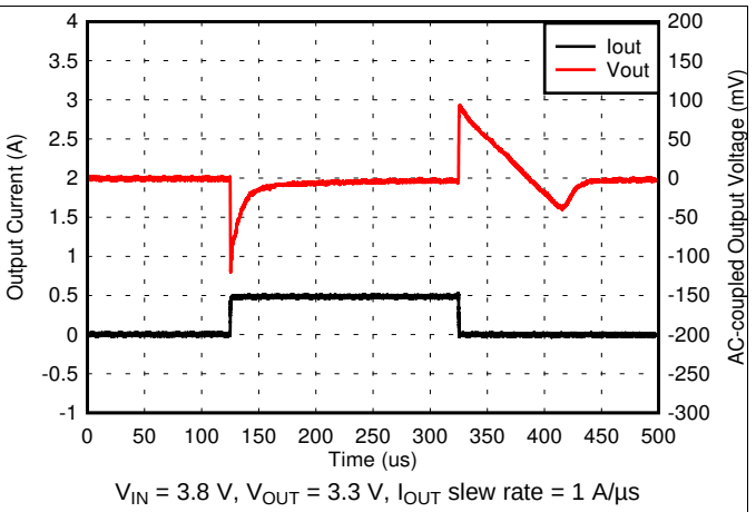
图 20. 3.3-V, 1-mA to 500-mA Load Transient
