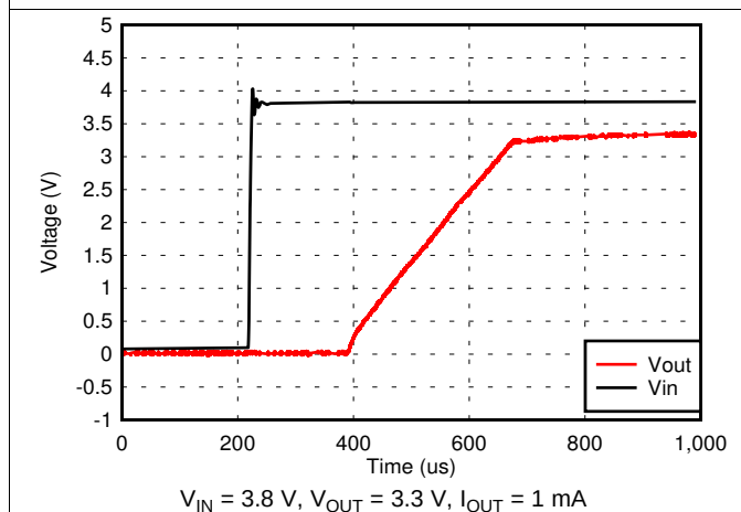
图 23. VIN Power-Up
