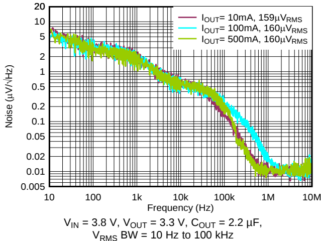
图 33. Output Spectral Noise Density
