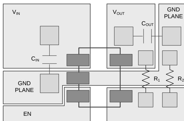
图 44. DBV Package Layout Example
