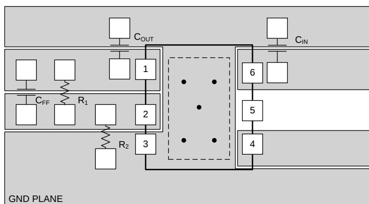
图 45. DRV Package Layout Example
