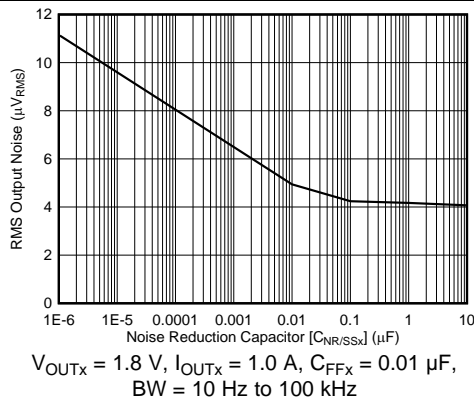
图 13. RMS Output Noise vs C_{NR/SSx}
