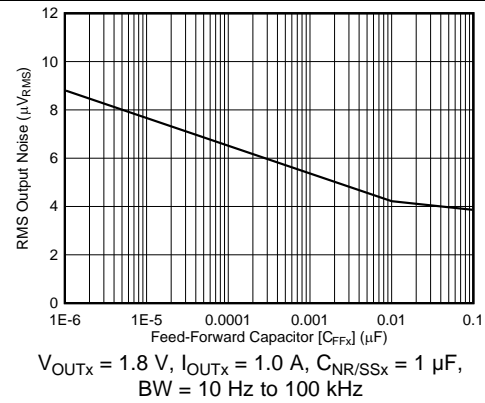
图 14. RMS Output Noise vs C_{FFx}
