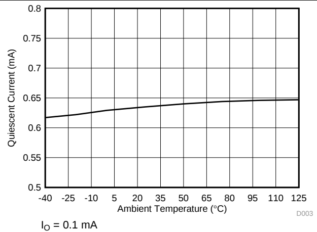
图 4. Quiescent Current vs Ambient Temperature (TPS7B7702-Q1)
