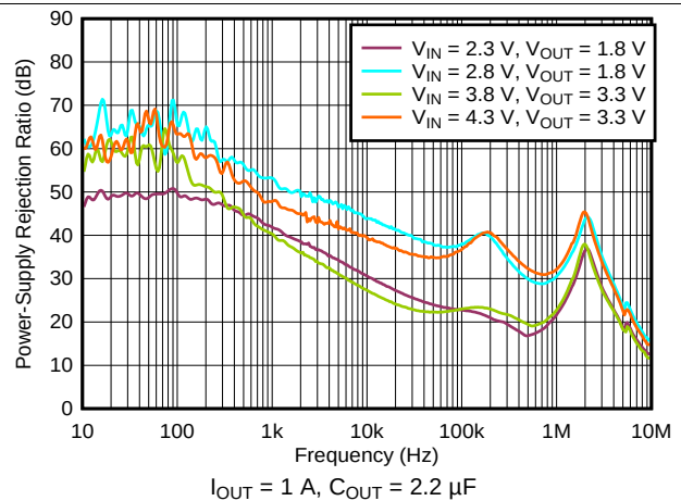
图 36. PSRR vs Frequency
