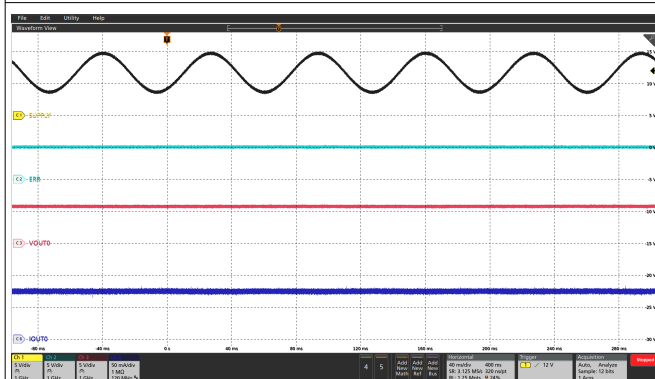
图 6-15. Transient Overvoltage
