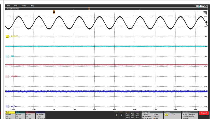
图 6-16. Jump Start
