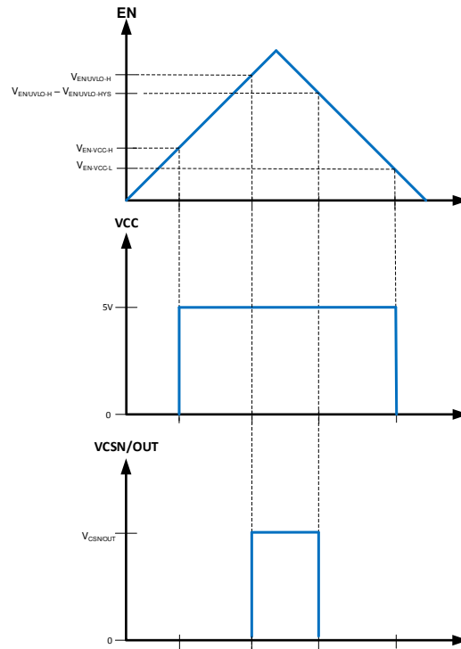
图 40. Precision Enable Behavior
