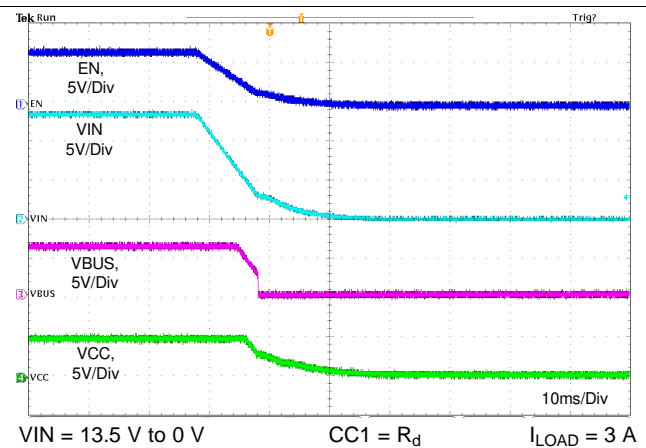
图 90. Shutdown Relate to VIN
