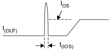
图 36. Short-Circuit Parameters
