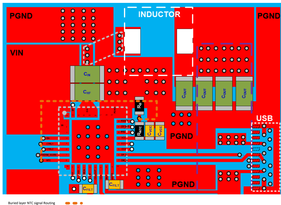
图 69. NTC Placement Example
