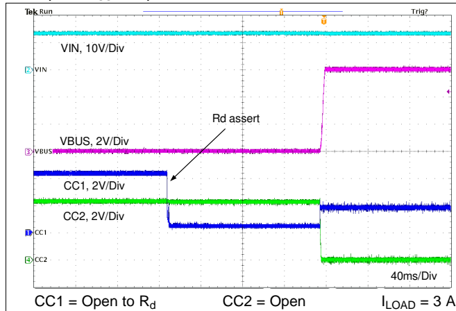
图 93. Rd Assert
