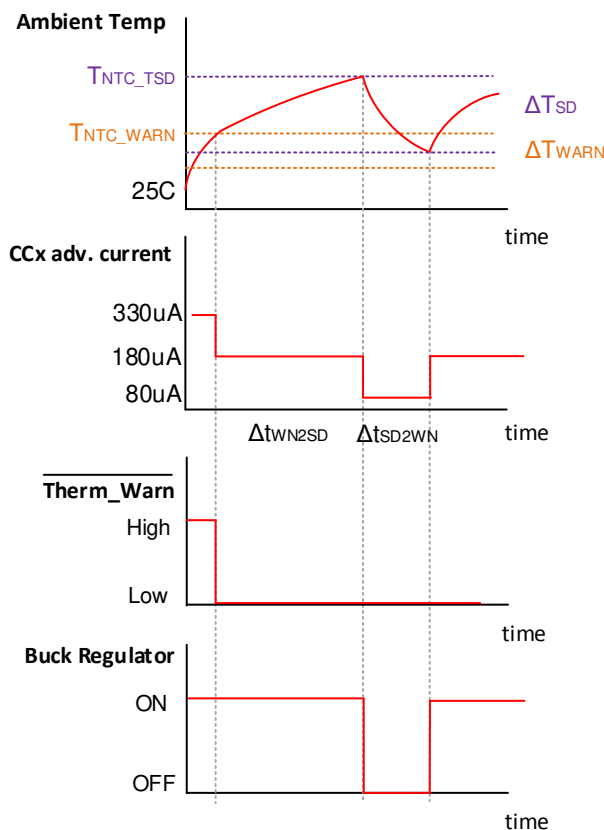
图 67. TPS25831-Q1 Behavior When Trigger NTC Threshold
