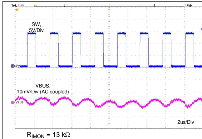
图 87. 100-mA Output Ripple
