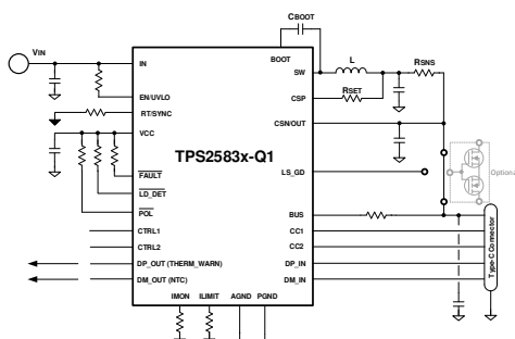
TPS2583x-Q1 简化原理图
