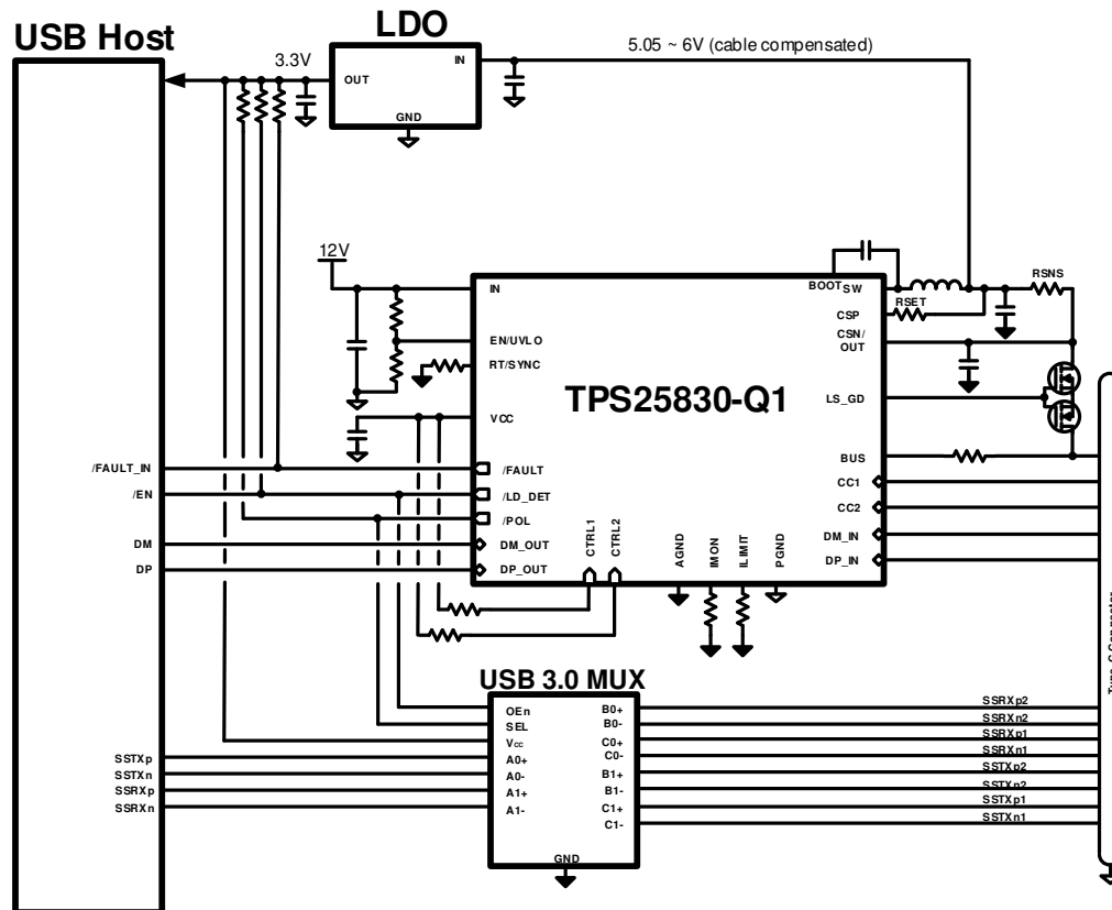
图 65. Example Implementation
