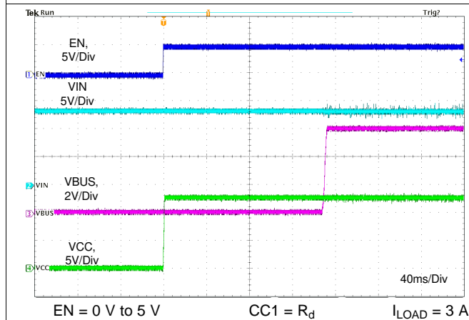
图 91. Startup Relate to EN
