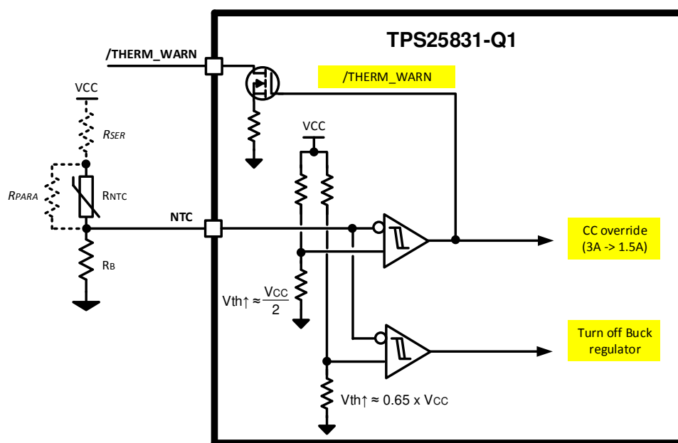
图 66. NTC Input Pin
