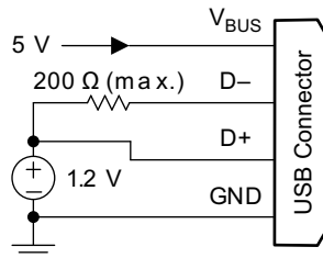
图 72. 1.2-V Mode
