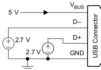
图 71. Divider 3 Mode
