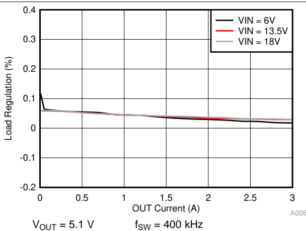
图 79. Load Regulation
