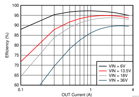
降压效率与输出电流间的关系 ( f_{\text{sw}} = 400\text{kHz} )
