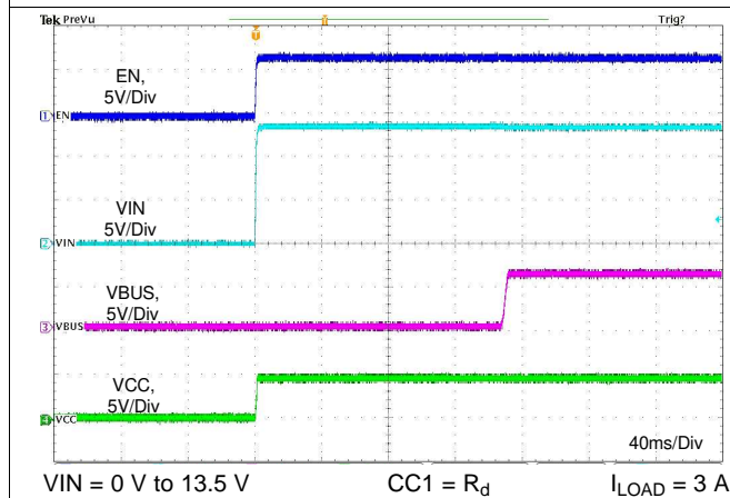
图 89. Startup Relate to VIN
