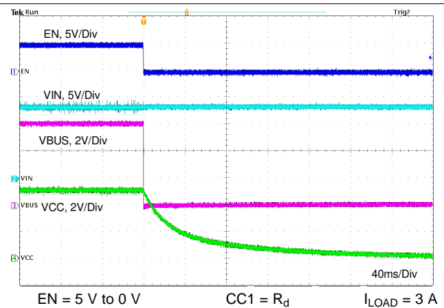
图 92. Shutdown Relate to EN
