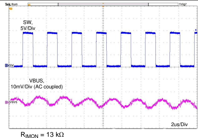
图 86. 3.5-A Output Ripple
