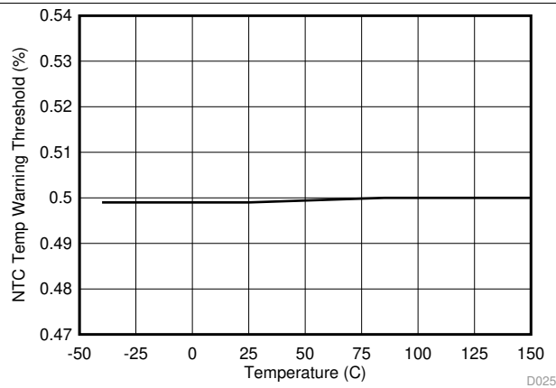
图 27. NTC Temperature Warning Threshold (TPS25831-Q1)
