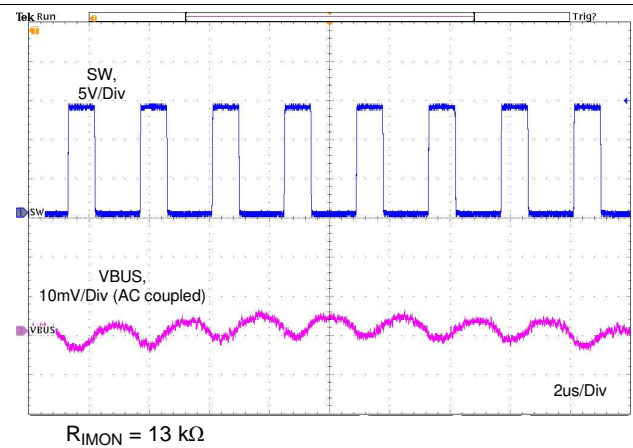
图 88. No Load Output Ripple
