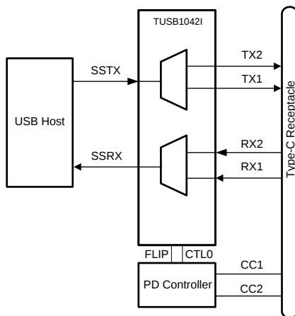
简化电路原理图
