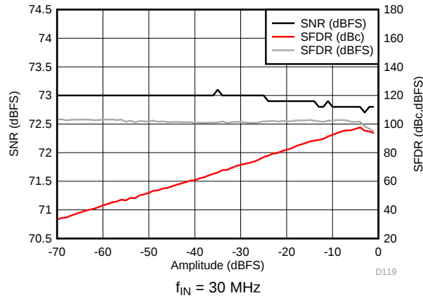
图 19. Performance vs Input Amplitude
