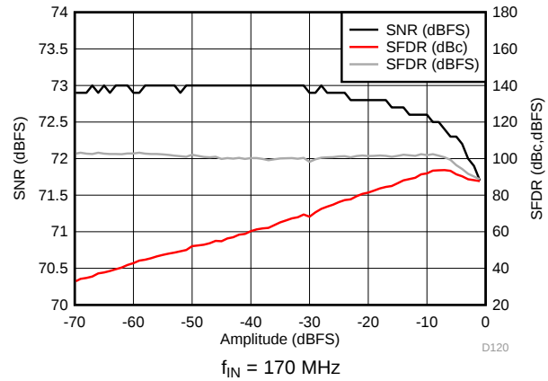
图 20. Performance vs Input Amplitude
