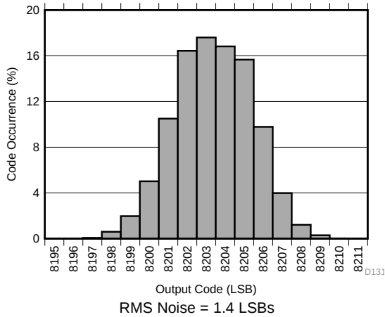
图 31. Idle Channel Histogram
