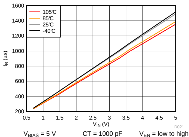
Figure 20. t_R vs V_{IN} , V_{BIAS} = 5\text{ V}
