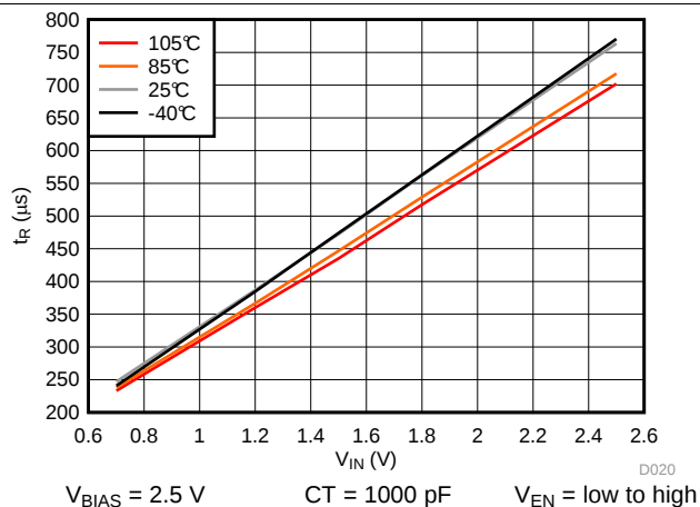
Figure 19. t_R vs V_{IN} , V_{BIAS} = 2.5\text{ V}
