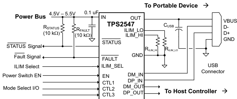
简化原理图
