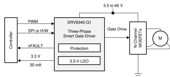
简化原理图
