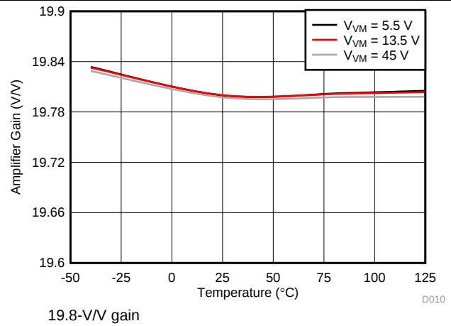
图 12. Amplifier Gain
