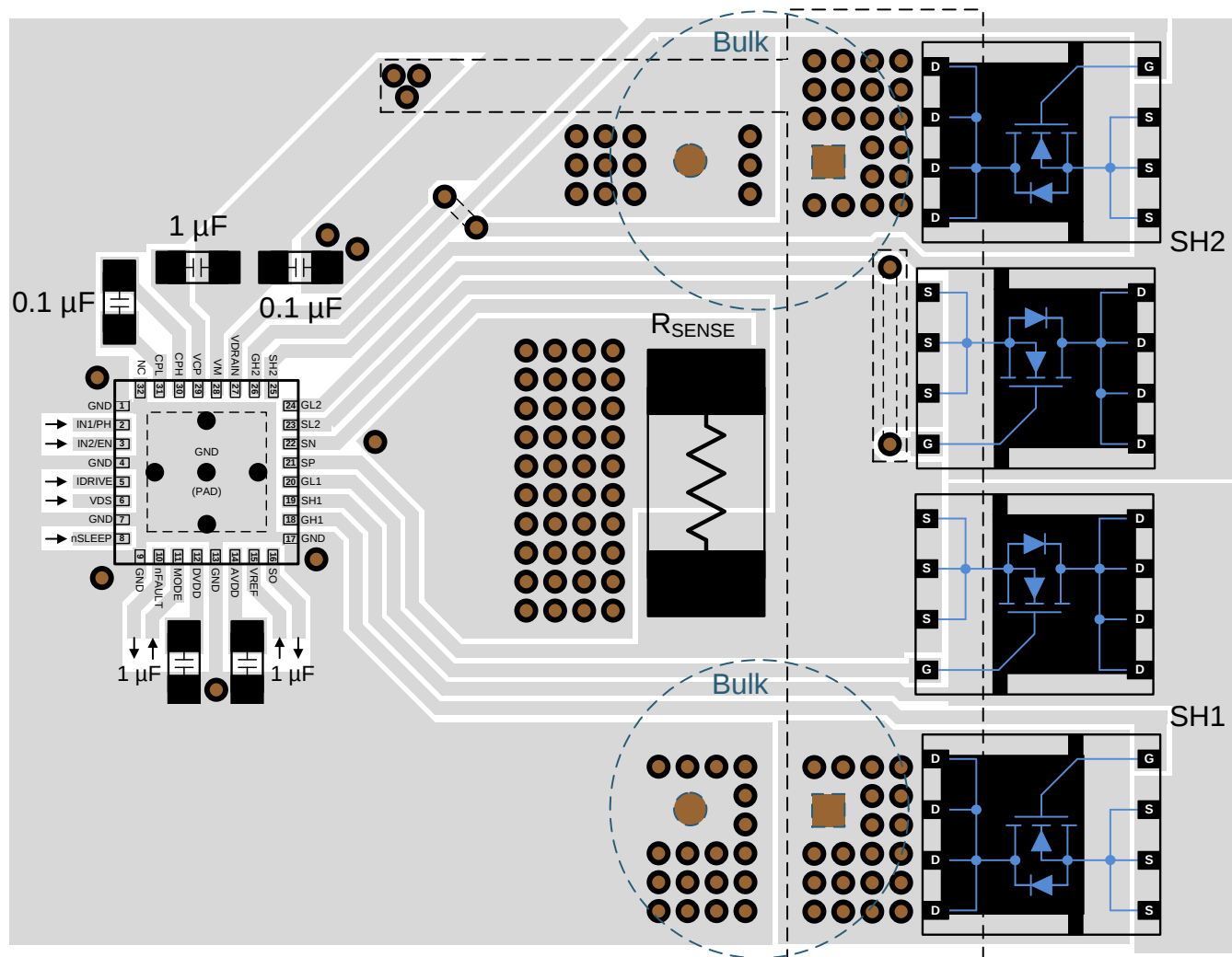
图 60. DRV8702-Q1 Layout Example
