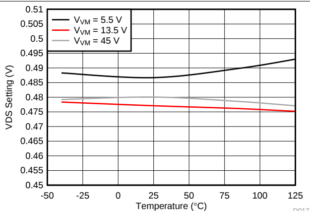
图 17. OCP Threshold Voltage
