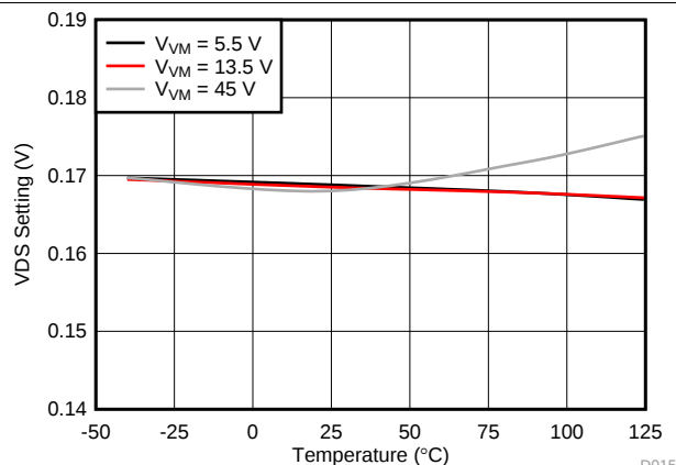
图 17. OCP Threshold Voltage
