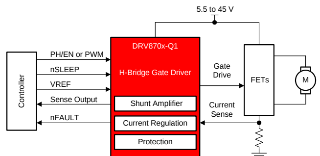
简化原理图
