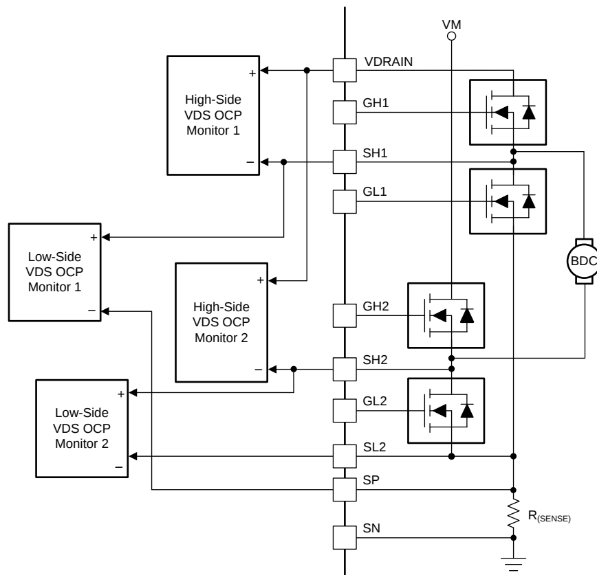
图 41. V_{DS(OC)} Block Diagram
