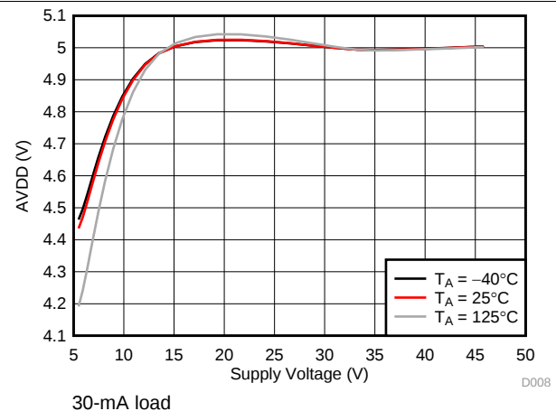
图 10. AVDD Regulator
