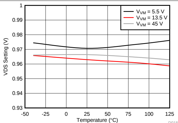
图 18. OCP Threshold Voltage
