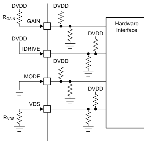
图 18. Hardware Interface
