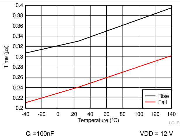
Figure 6-20. LO Rise & Fall Time
