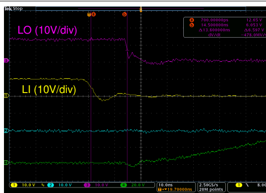
Figure 8-6. LO Fall Time
