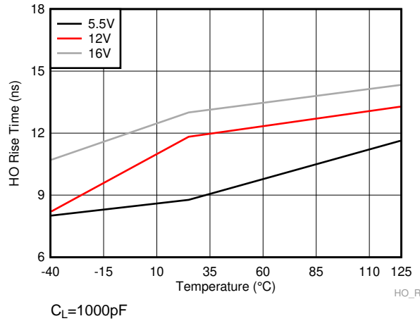
图 18. HO Rise Time
