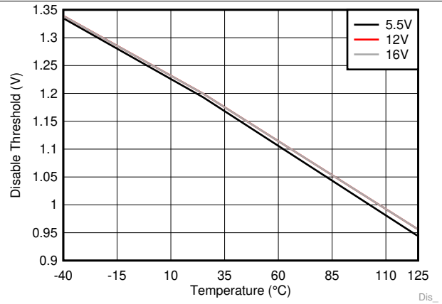
图 11. Disable Threshold
