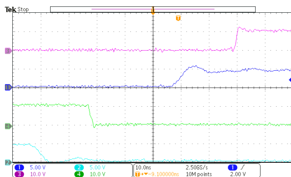
图 29. LO Fall Time
