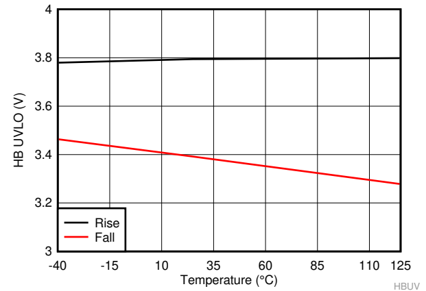
图 11. Disable Threshold
