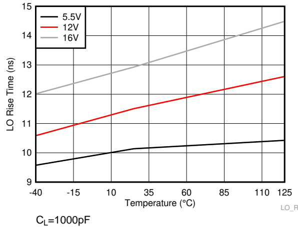
图 16. LO Rise Time
