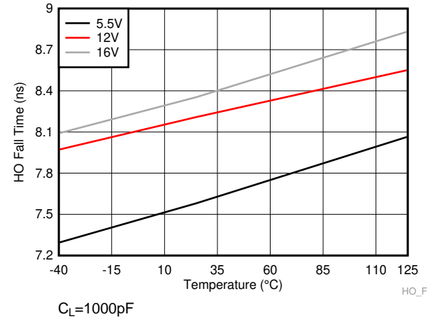
图 19. HO Fall Time
