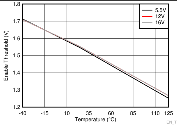
图 10. Enable Threshold
