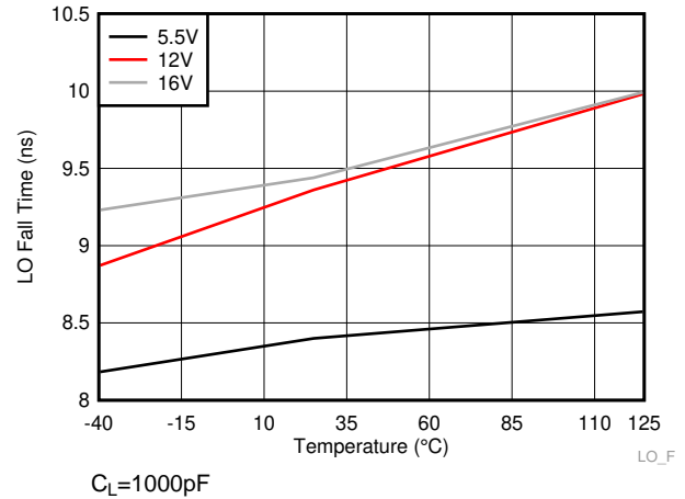
图 17. LO Fall Time
