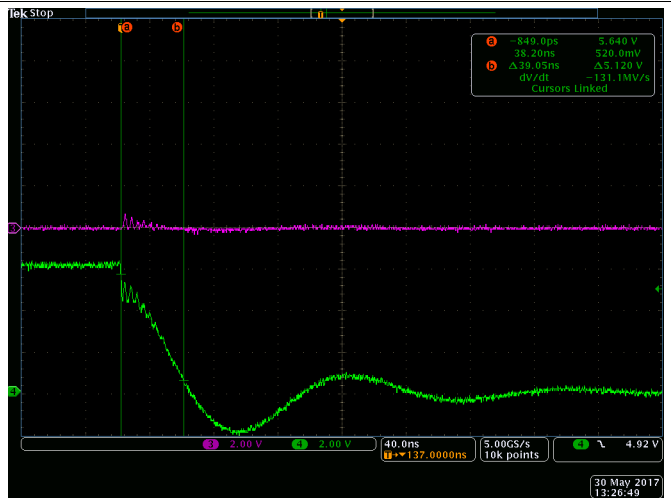
图 39. LO Fall Time
