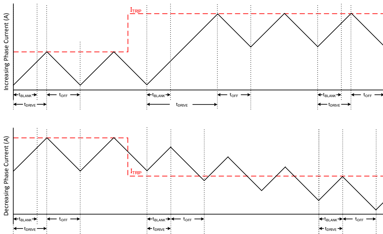
图 7-7. 快速/快速衰减模式
