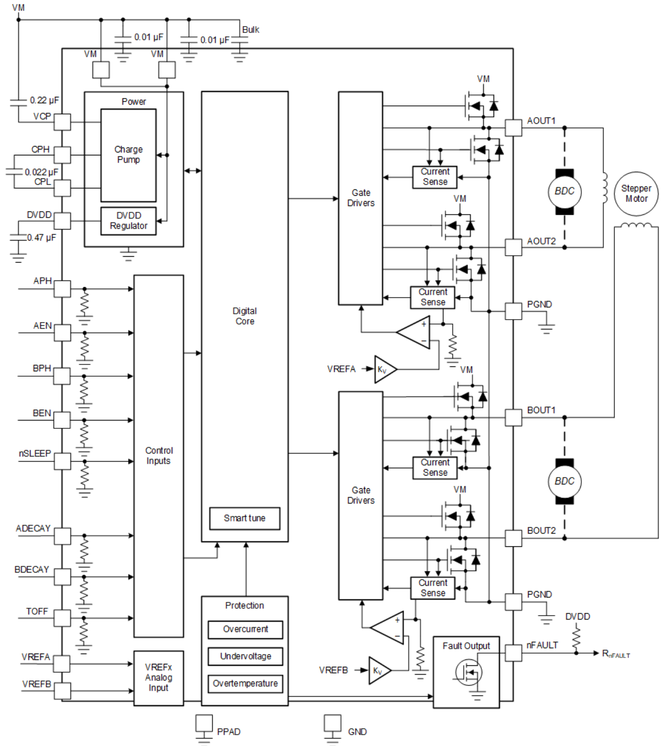
图 7-1. DRV8426E 方框图
