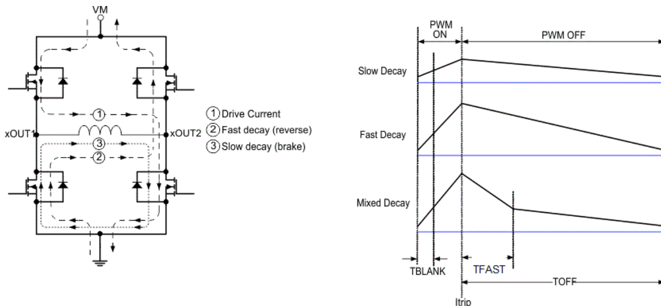
图 7-5. 衰减模式
