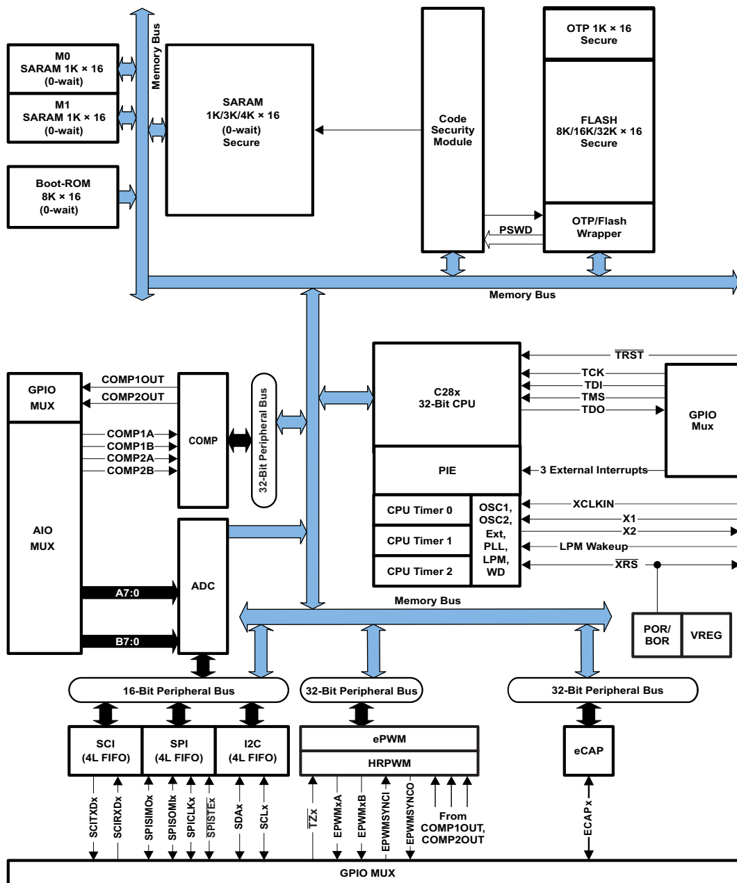
图 1-1. 功能方框图
