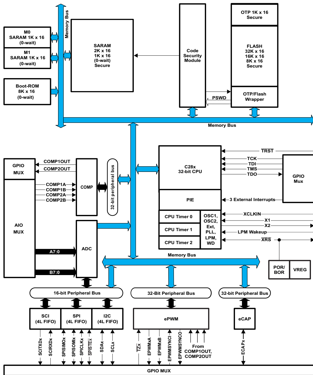
图 1-1. 功能框图
