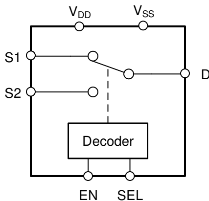
TMUX6219 方框图
