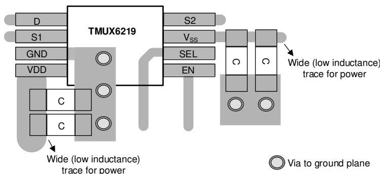
图 11-2. TMUX6219 Layout Example
