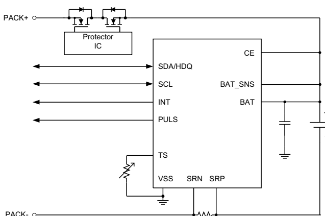
简化原理图
