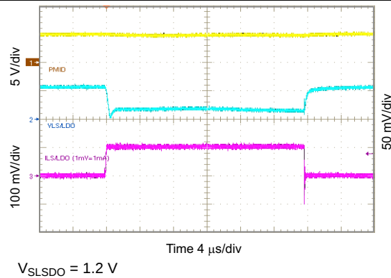
图 89. 1.2 V_{SLSDO} Load Transient, 0 to 100 mA
