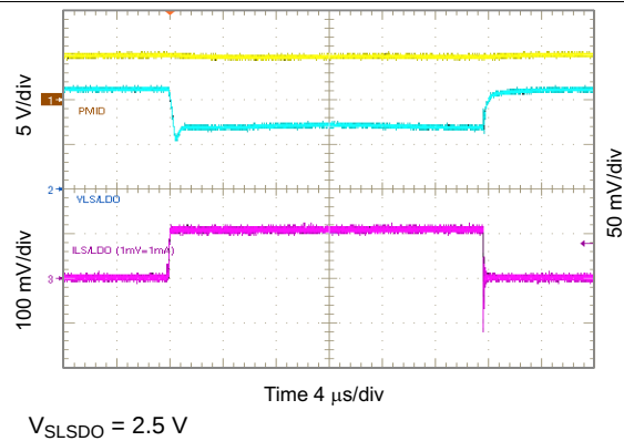
图 91. 2.5 V_{SLSDO} Load Transient, 0 to 100 mA
