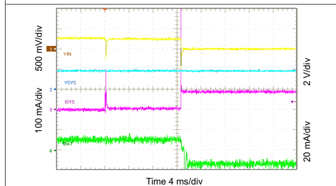
图 40. Entering DPPM Mode
