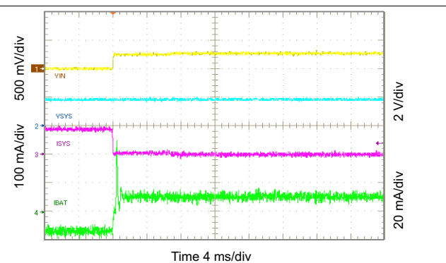
图 41. Exiting DPPM Mode
