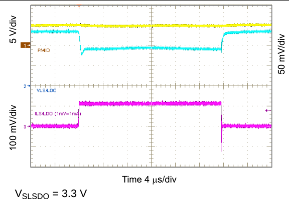
图 92. 3.3 V_{SLSDO} Load Transient, 0 to 100 mA
