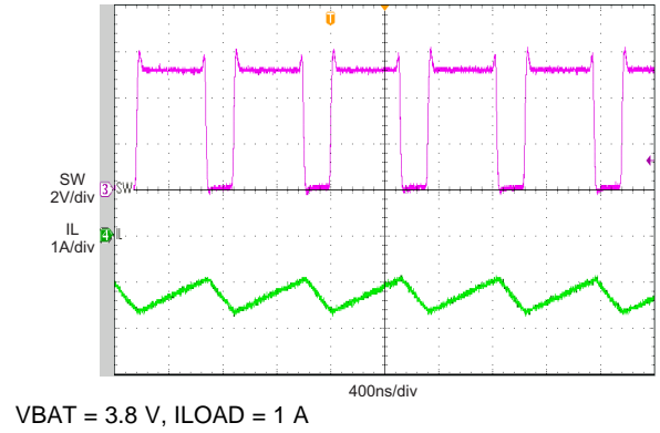
图 46. Boost Mode Switching
