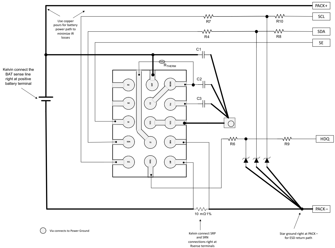
图 14. Layout Example
