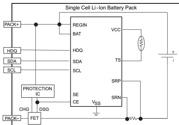
简化原理图
