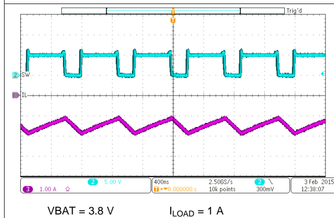
图 56. PWM Switching Waveform
