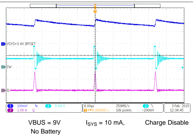
图 57. PFM Switching Waveform
