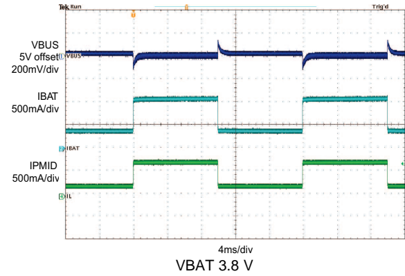
图 41. Boost Mode Load Transient
