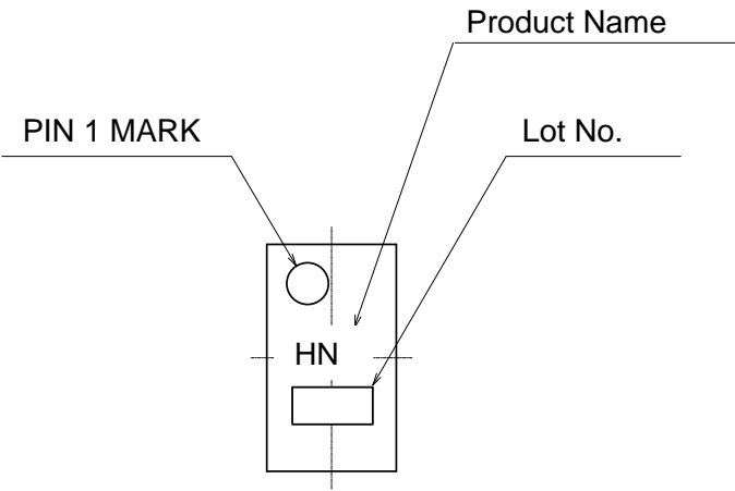
UCSP30L1A (BU64981AGWZ)
