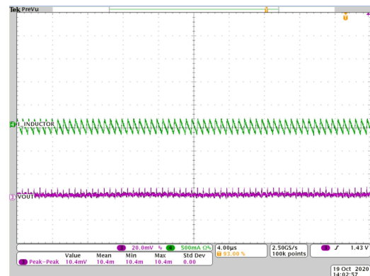
图 8-44. Output Voltage Ripple
