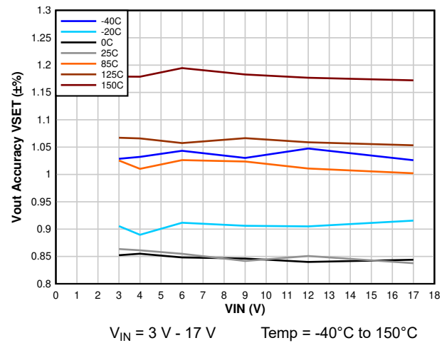
图 8-67. Output Voltage Accuracy - VSET Selected
