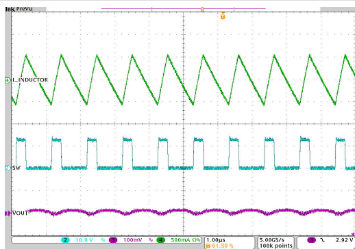
图 8-49. Output Voltage Ripple
