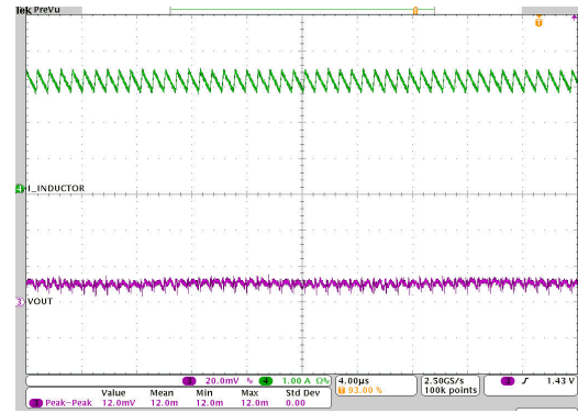
图 8-48. Output Voltage Ripple
