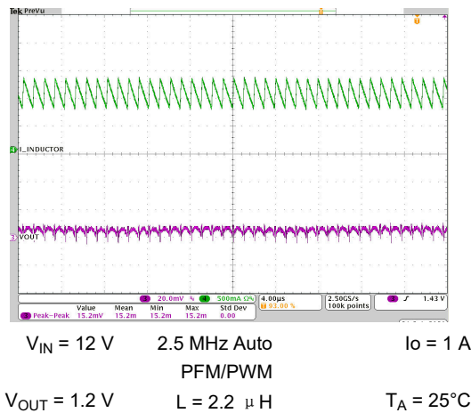
图 8-66. Output Voltage Ripple
