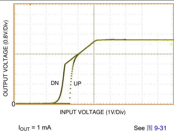
图 7-5. UVLO Thresholds
