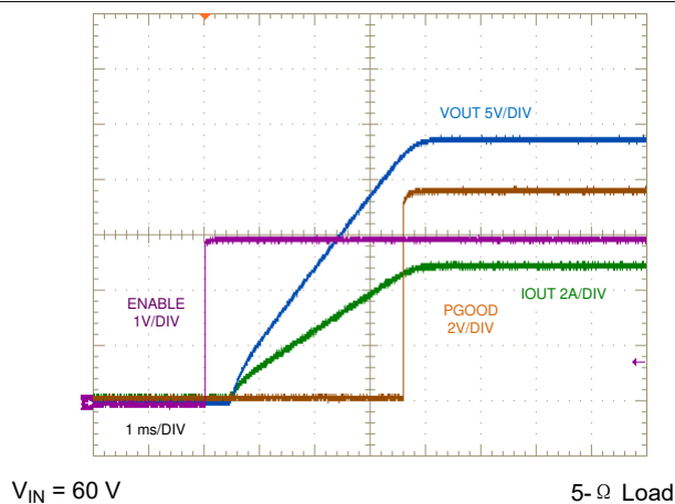
图 9-38. ENABLE ON, 5-A Resistive Load
