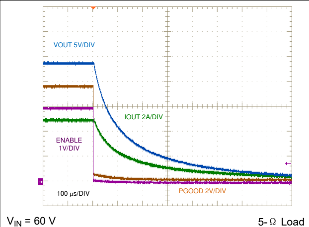
图 9-39. ENABLE OFF, 10-A Resistive Load
