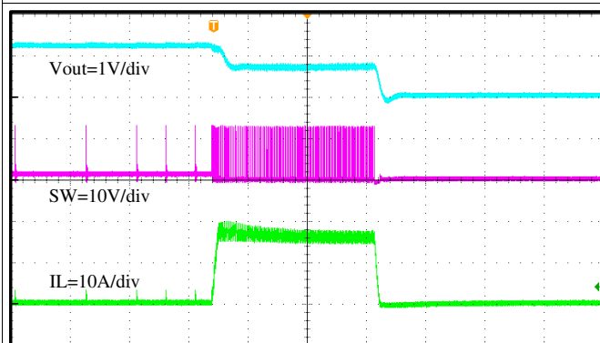
图 31. Transient Response
