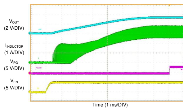
图 56. LM61440-Q1 Start-up with 3.25-A
