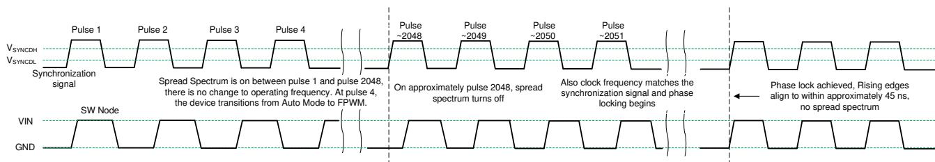
图 12. Synchronization Process
