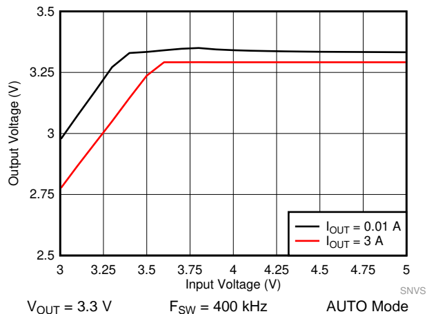
图 46. LM61440-Q1 Dropout Curve
