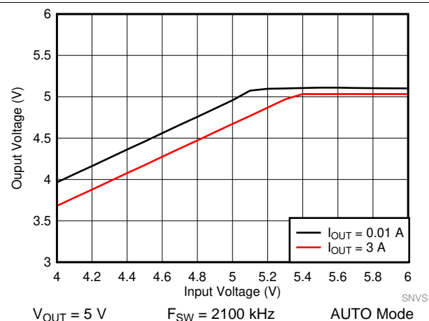
图 49. LM61440-Q1 Dropout Curve
