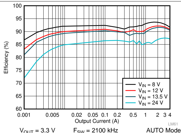
图 34. LM61440-Q1 Efficiency
