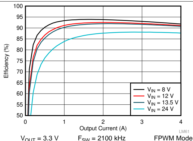
图 35. LM61440-Q1 Efficiency
