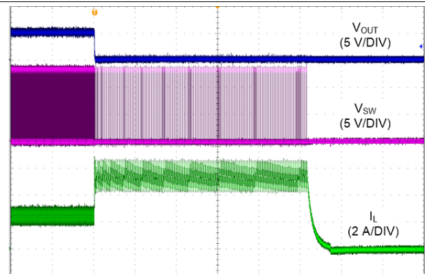
图 57. LM61440-Q1 Short Circuit Protection
