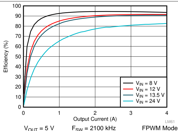
图 37. LM61440-Q1 Efficiency
