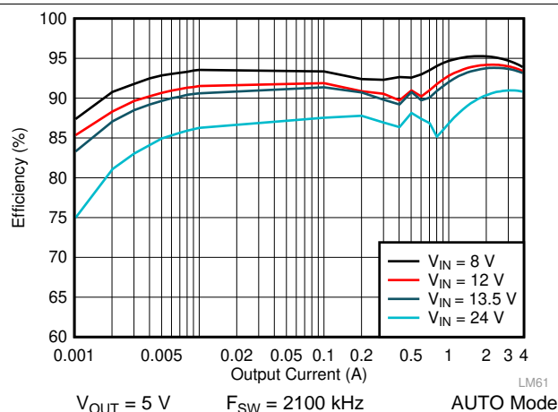
图 36. LM61440-Q1 Efficiency
