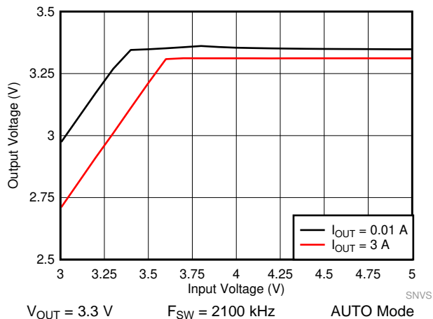
图 47. LM61440-Q1 Dropout Curve
